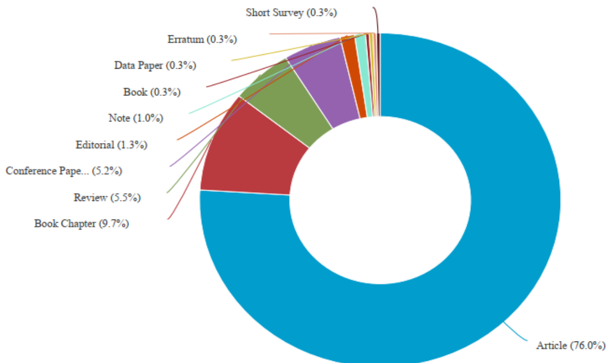
Рис. 3. Розподіл за типом проіндексованих у Scopus публікацій, які містять у назві, анотації, ключових словах термін «land degradation neutrality», 2015–2023 рр.
